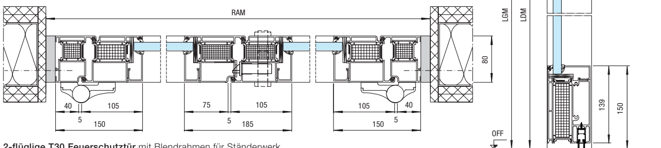
2-flüglige T30 Feuerschutztür mit Blendrahmen für Ständerwerk
