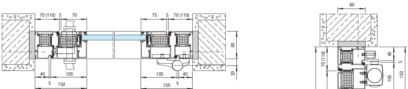
1-flüglige T30 Feuerschutztür mit Blendrahmen für Mauerwerk
