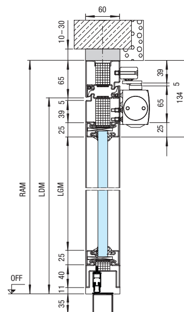
1- / 2-flügelige T30 Stahl-Feuerschutztür S-Line mit Blendrahmen für Mauerwerk
